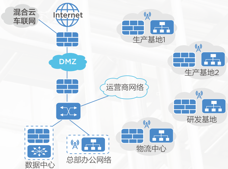
图 12 初创期网络建设方案
