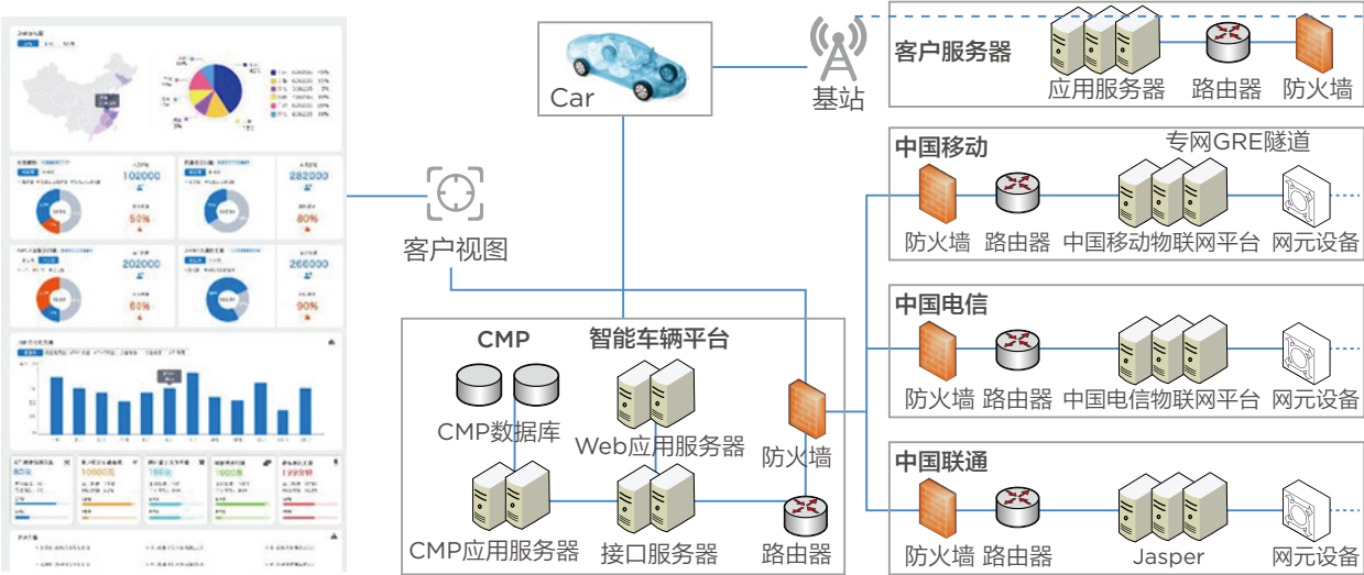
图 19 联想车联网方案——智能连接管理平台
