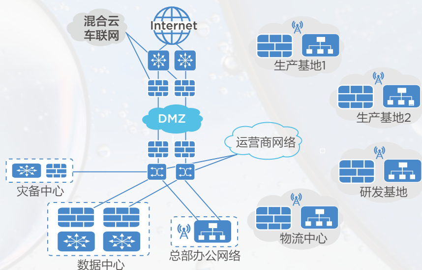
图 16 成长期网络规划方案
